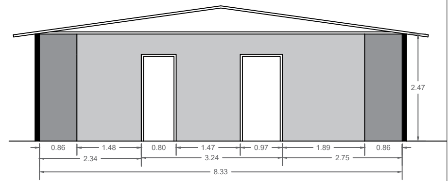
CORTE B-B'
